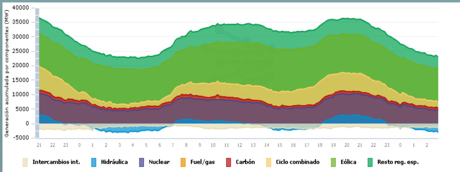
Detalle de la estructura de generación en tiempo real
