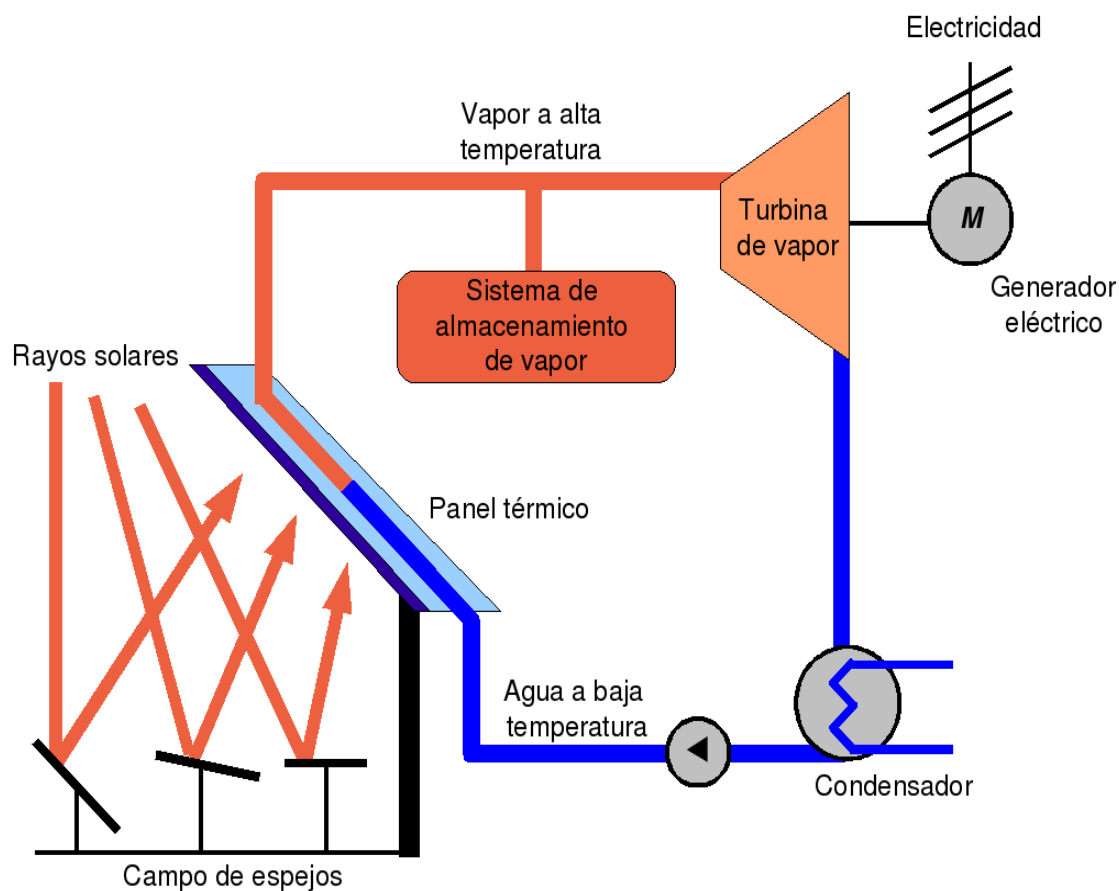
PS-20 (Sevilla). 20 MW
