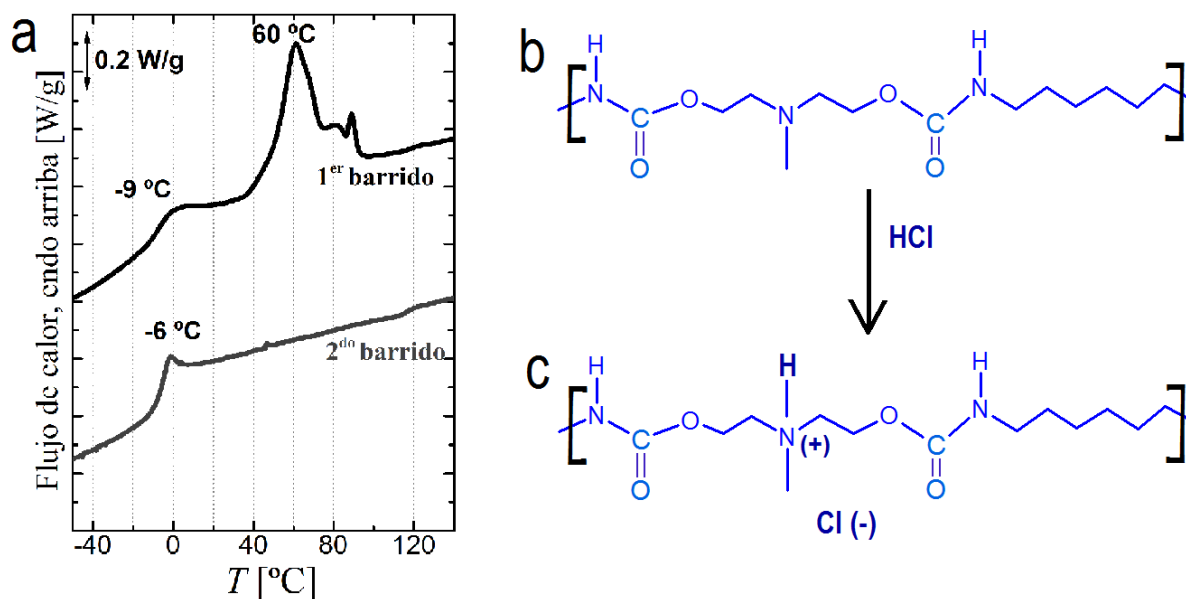
Figura 1. a) Caracterización térmica del poliuretano tras 4 horas/100°C, enfriamiento lento y mantenido 10 horas a temperatura ambiente (1er barrido); y termograma del segundo barrido, tras un enfriamiento desde el fundido a 20°C/min y mantenido 1 minuto a -60°C. b) Estructura del poliuretano estudiado y b) su solubilización tras la cuaternización con HCl.
