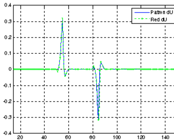
Fig. 4. Salida devuelta por la red ante un conjunto de patrones que recogen como consigna un pulso ideal. Dicho conjunto fue utilizado en el proceso de entrenamiento.
