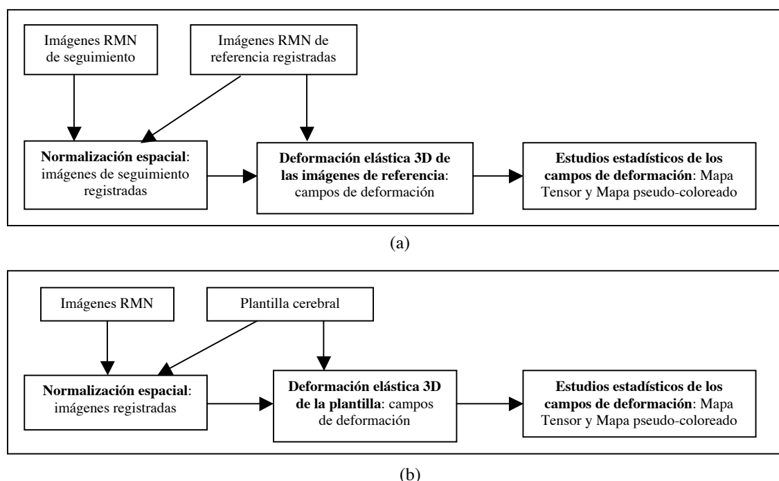
Figura 3. Diagrama de flujo genérico de los métodos TBM en un estudio longitudinal (a) y en un estudio transversal (b).
