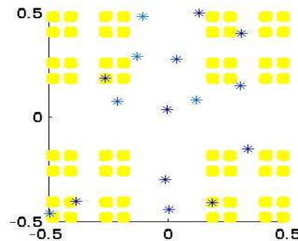
Figura 1: Representación del conjunto de Cantor (·) y del codebook inicial (*) generado aleatoriamente, solo se muestran la 2º y 4º dimensión.
