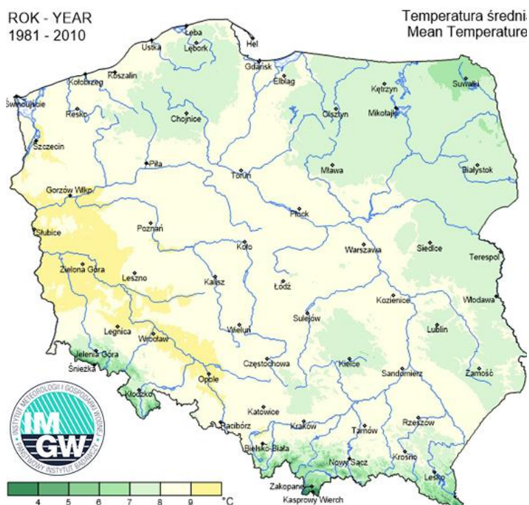
Irudia 6-1. Poloniako batz besteko temperaturak .
