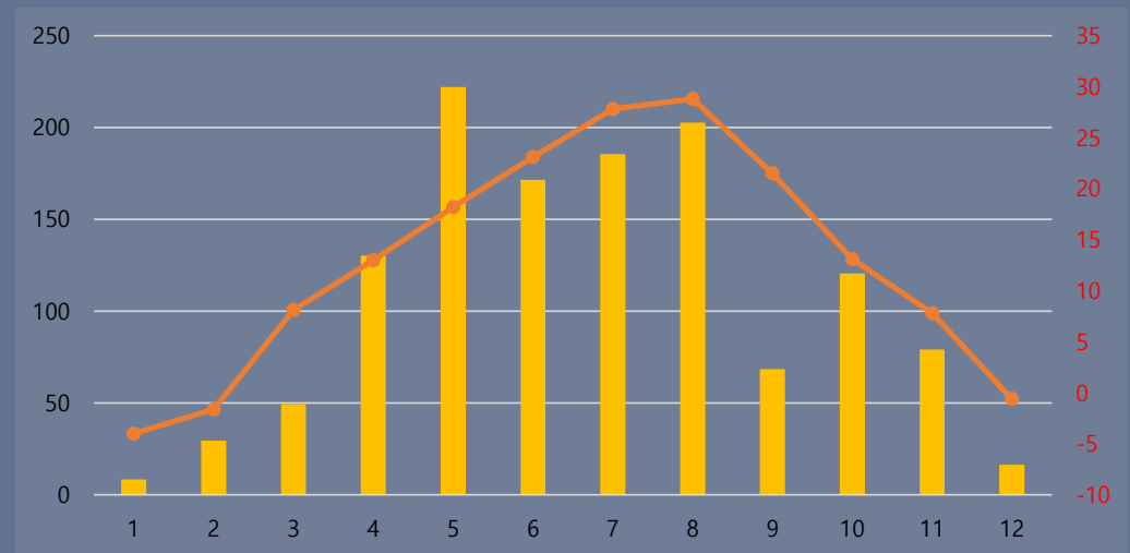
Rainfall(mm) Temperature(°C)
