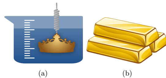
Figura 1: Aparato utilizado para la medición de la masa aparente. En la figura a) se muestra su uso para la corona, en la figura b) se muestran los lingotes de oro usados de referencia.
