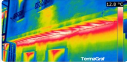
Vitoria-Gasteizko Ingeniaritza Eskolan klimatizazioarako energia kontsumoa optimizatzea
