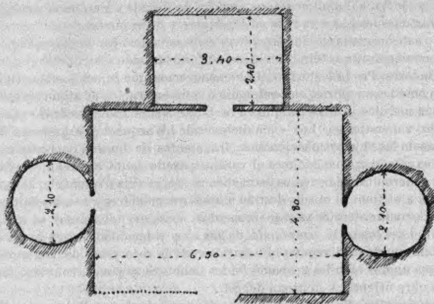
(Fig. 24).—Croquis en planta de una de las cuevas artificiales situadas al N. de Laño
