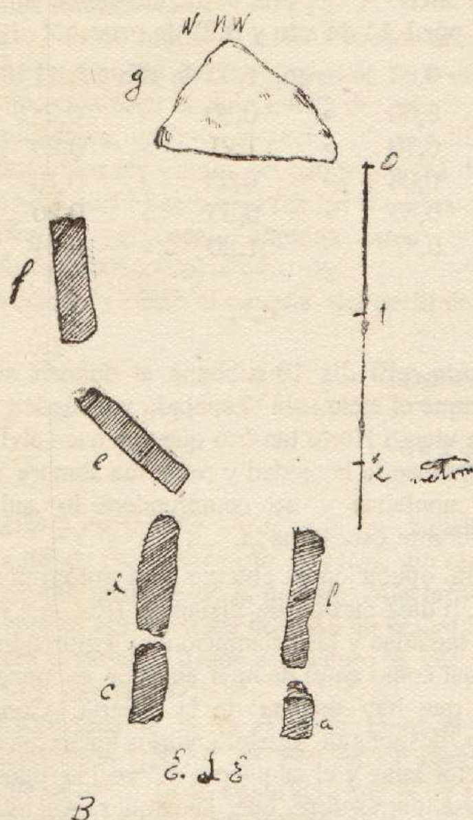
(Fig. 7. a ) Igartza occidental.—B. Planta del dolmen
