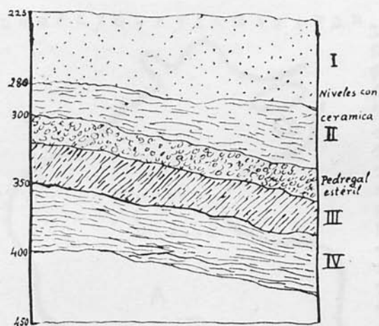
FIG. 3.—LUMENTXA. Corte del yacimiento en 1 c - 25 c.
